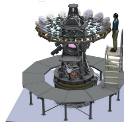
Diseño detallado del telescopio MiniELF.
