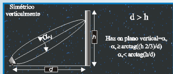
Gráficos de utilización de proyectores simétricos en función del haz luminoso y la distancia al objeto a iluminar.
