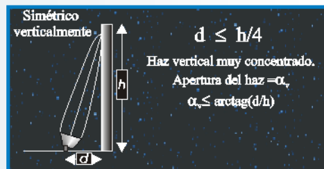
Gráficos de utilización de proyectores simétricos en función del haz luminoso y la distancia al objeto a iluminar.
