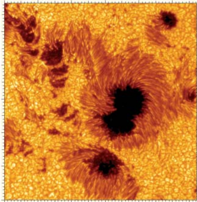
Figura 6a. Mancha solar obtenida con el Telescopio Solar Sueco en el Observatorio del Roque de los Muchachos - Garafía - La Palma.
