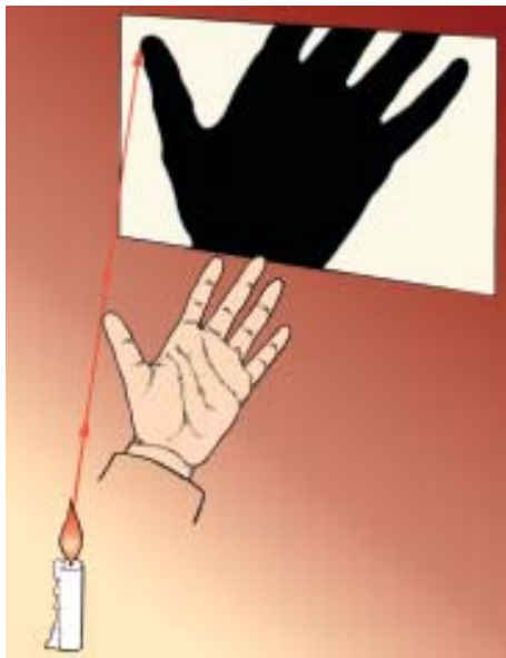
Figura 3. Proyección de sombras.
