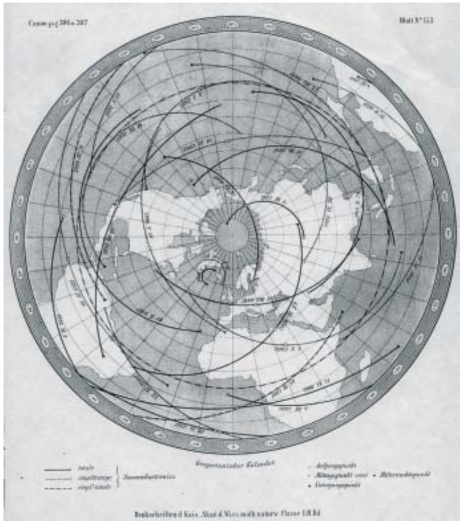
Figura 10. Un mapa del Canon de Oppolzer, que muestra la línea central de los eclipses solares entre el 19 de mayo de 1985 y el 7 de febrero de 2008. Los eclipses totales aparecen como líneas continuas y los anulares, como líneas de trazos. Nótese que algunas líneas de centralidad pueden mostrar discrepancias con mapas modernos. Esto es debido a que el trazado de dichas líneas se realizó calculando solo tres puntos que se unieron con un arco circular. Para un cálculo exacto el propio Oppolzer recomendó utilizar las tablas numéricas del Canon.
