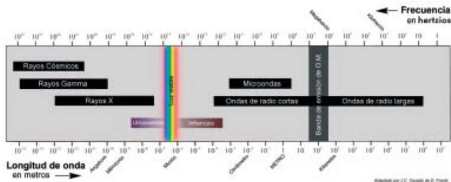
Figura 1. La luz visible en el espectro electromagn3tico.
