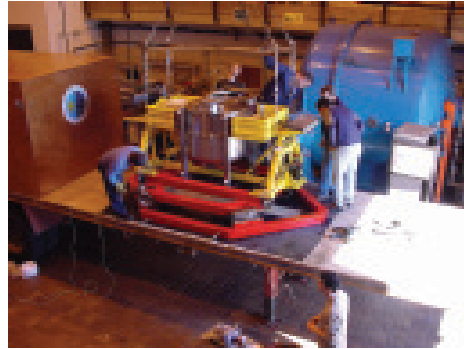
LIRIS integrado sobre el útil de transporte (estructura roja).
