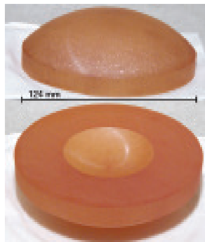
2 vistas del blanco de ZnSe que servirá, tras los ensayos, para pulir la sexta lente de cámara de EMIR.
