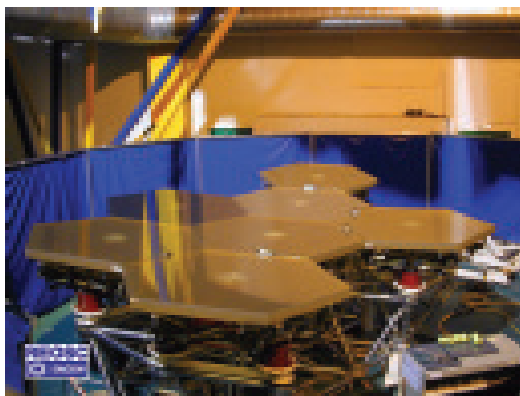
Segmentos del espejo primario del GTC montados en asociación junto al segmento maestro para su pulido.
