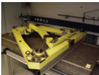
Subsistema del colimador del instrumento OSIRIS.
