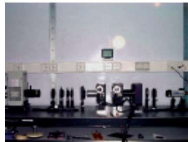
IAC: Banco óptico para caracterización de los ROCLIs.
