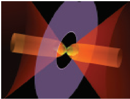
Modelo que reproduce las características morfológicas y cinemáticas de las cuatro componentes de Mz-3: Lóbulos centrales, columnas, conos bipolares y disco.
