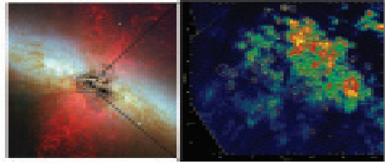
Imagen de la galaxia M82 (estructura azulada con forma de puro) y la superposición en rojo de los filamentos (supervientos galácticos) obtenidos con un filtro que mide al gas ionizado, por el telescopio de 8 m SUBARU. El cuadrado superpuesto en la parte central es el campo observado con el telescopio espacial HST. En la imagen de la derecha se presenta parte de ese campo del HST con los supercúmulos que se han identificado y catalogado, del análisis de las imágenes disponibles en el archivo. En un área de 250x250 pc se identificaron 199 SSCs (Melo et al.).
