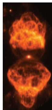
Imagen HST de la zona central de la Nebulosa Planetaria Mz-3, tomada con un filtro estrecho en H\alpha+[NII] por R. Corradi y colaboradores.
