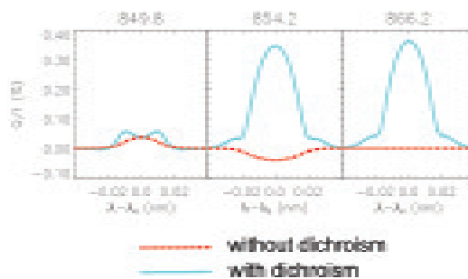
Dicroísmo a campo nulo en la cromosfera solar: Polarización lineal del triplete infrarrojo del calcio ionizado calculada en un modelo empírico de la atmósfera solar teniendo en cuenta todos los mecanismos de bombeo radiativo en un modelo atómico realista. Las líneas azules muestran los perfiles Q/I emergentes cuando se tiene en cuenta la absorción diferencial producida por la polarización atómica de los niveles inferiores de dicho triplete. Los perfiles de polarización calculados y sus amplitudes relativas están de acuerdo con las observaciones. Las líneas en color rojo indican los perfiles Q/I que resultan si se supone que los subniveles de dichos niveles inferiores están todos igualmente poblados.
