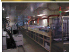
Instalaciones de Tecdis. Arriba: línea de fotoexposición. Izquierda: línea de ataque ácido.
