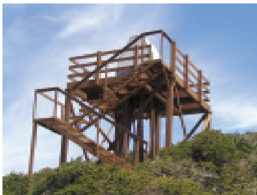
Vista del actual monitor de seeing DIMM desarrollado por el IAC.
