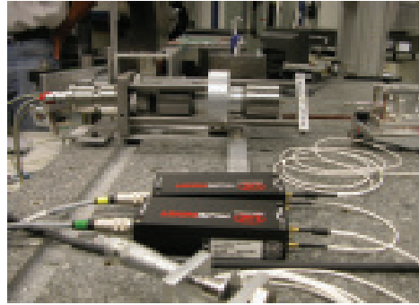
Foto 2. Uno de los actuadores del colimador en fase de montaje
