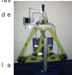
Foto 3. Soporte del Colimador
