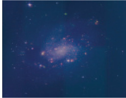
Foto superior: imagen de la galaxia del Grupo Local NGC 300 en filtros que aíslan la emisión en [OIII] (verde), H- \alpha más [NII] (rojo) y el continuo (azul). Las nebulosas planetarias y otras nebulosas de alta excitación aparecen en amarillo y verde, las regiones HII en rojo y las estrellas en blanco. Imágenes tomadas en el telescopio de 2.2 m de la ESO por P. Leisy.
