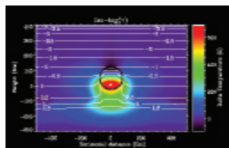
Mapa de la diferencia de temperatura de un tubo penumbral y su entorno respecto al modelo sin tubo, para el caso de un tubo de 75 km de radio, con un campo magnético 500 G mayor que el entorno y una inclinación 45° mayor que la del entorno. El eje del tubo está situado a 50 km por encima de la capa de profundidad óptica unidad en el continuo a 5.000 Å. Los contornos corresponden a las isolíneas en profundidad óptica. El exceso de temperatura en la parte inferior del tubo alcanza los 680 K mientras que el déficit en la zona de sombra (parte superior del tubo) alcanza -40 K. La temperatura efectiva del modelo penumbral en calma es de 4.790 K.
