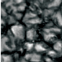
Imagen de granulación solar (17.4"x17.4") obtenida el 30 de septiembre de 2003, en el telescopio SST (ORM, La Palma). Esta imagen resulta de la restauración y combinación de 4 imágenes individuales tratadas con la técnica de Diversidad de Fase.
