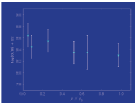
Primer gradiente de abundancias estelares obtenido más allá del Grupo Local. Se presenta el gradiente de O en NGC 300.
