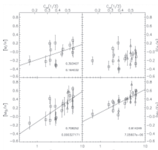
Representación de la metalicidad global [M/H] , [Fe/H] , y [Mg/H] y de la razón de abundancias [Mg/Fe] frente a los parámetros de forma n y C_v(1/3) . Las galaxias del cúmulo de Virgo se representan por cuadrados mientras que las de campo se representan por triángulos. Los coeficientes de correlación de Spearman y su representatividad están indicados en cada gráfico.
