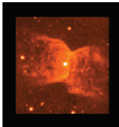
Imagen de la nebulosa planetaria NGC 2346 en la línea de hidrógeno molecular H_2 v=1-0S(1) en 2,122 micras. El tamaño de la imagen es de 3,2x2,8 minutos de arco. La estructura en forma de grumos y la estrella central sólo son visibles en infrarrojo. El Norte está a la derecha y el Este arriba.
