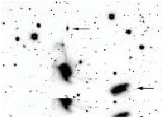
Imagen profunda en el filtro R de la galaxia Mrk 1087 y sus alrededores (obtenida con el telescopio NOT, del ORM). Presenta una gran cantidad de estructuras posiblemente producidas por interacción con otras galaxias independientes de los alrededores, localizadas justo al Norte y al Oeste-Suroeste de Mrk 1087 (indicadas en la figura). También se observa un racimo de galaxias enanas de marea nacidas posiblemente a partir de material expulsado de la galaxia principal.
