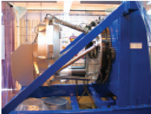
El instrumento ELMER, en los talleres del IAC, instalado en su banco de pruebas.
