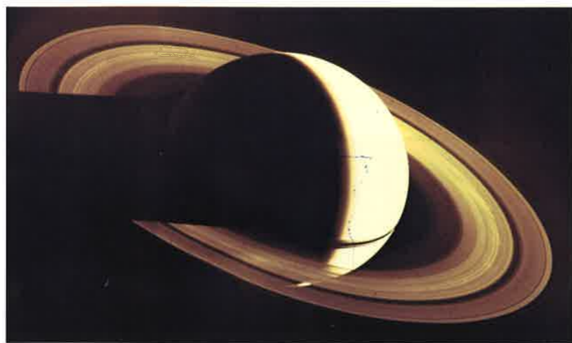
Saturno, fotografiado por Voyager 2, cuando partía hacia Urano. © NASA.
