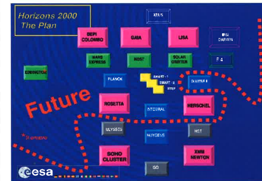
Figura 1. Esquema del antiguo programa científico de la ESA Horizon 2000+ que ha sido recientemente reestructurado y ampliado en Cosmic Vision 2020.
